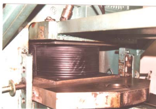
Essai de Compression sur isolateur
